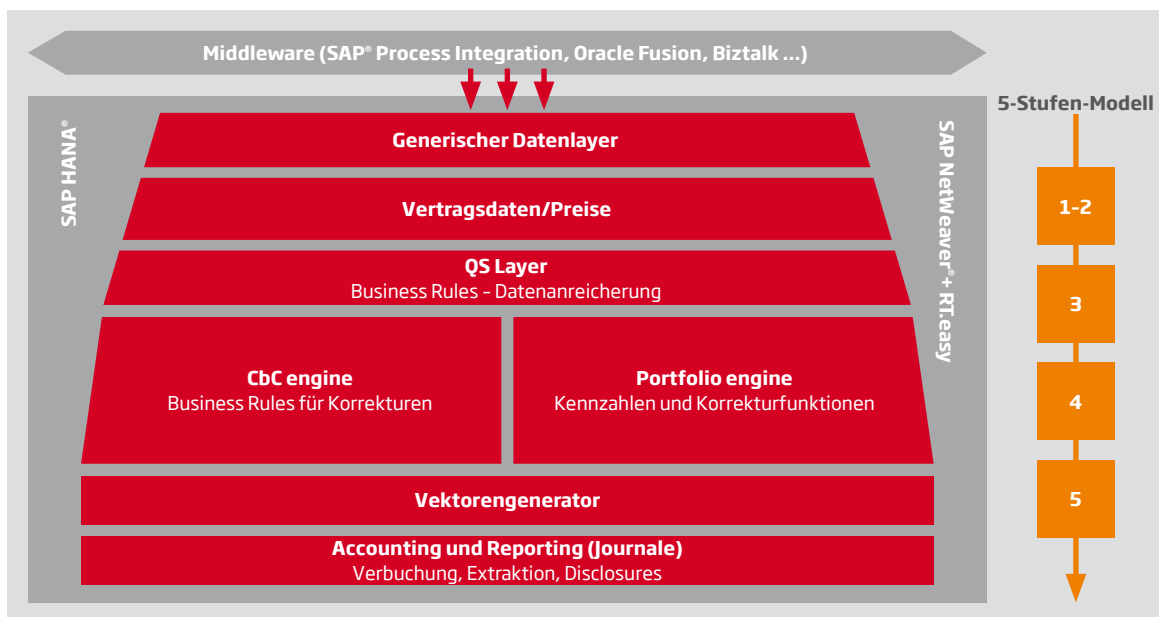
Abb. 2: Architektur IFRS15.easy
